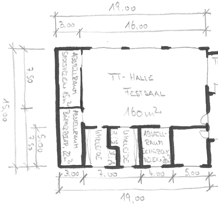
GRUNDRISS ERDGESCHOSS
